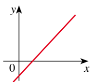
Graf rastúcej funkcie
