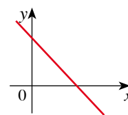
Graf klesajúcej funkcie
